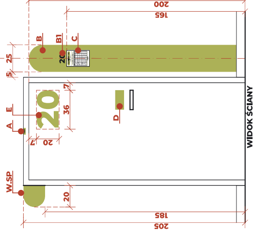
W.DO_02 - DRZWI DO POMIESZCZENIA OGÓLNEGO
