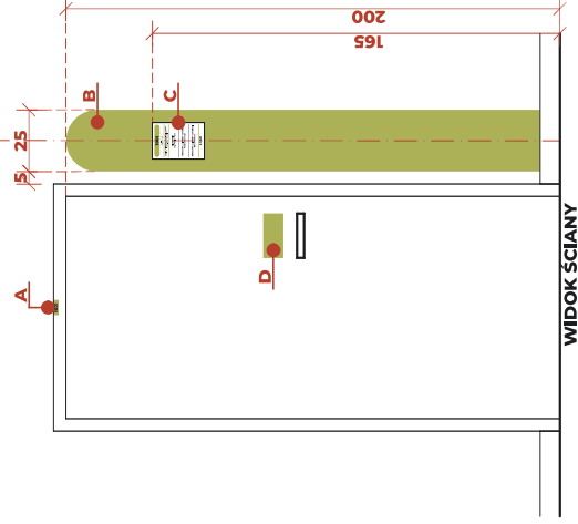
W.DO_01 - DRZWI DO POMIESZCZENIA OGÓLNEGO
